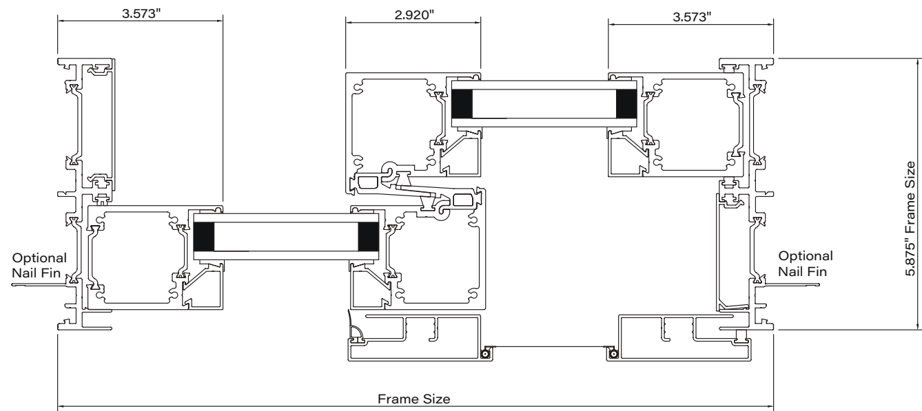
7650 XO condition
