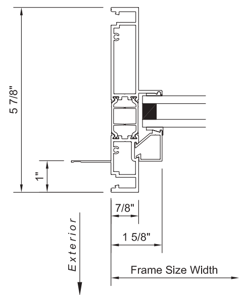
jamb nail fin frame
