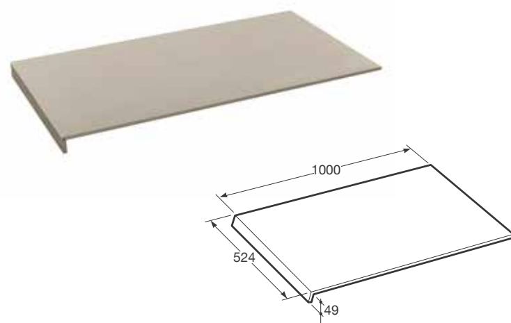
L1 GREIGE CANNETÉE R 4,9 x 100.
