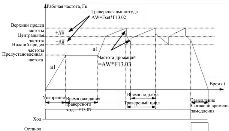
Рис.7-43 Трассовый ход
