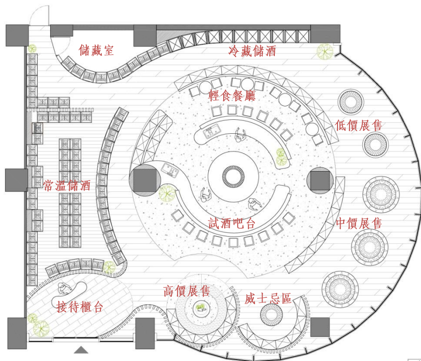
平面配置圖S:1/100
