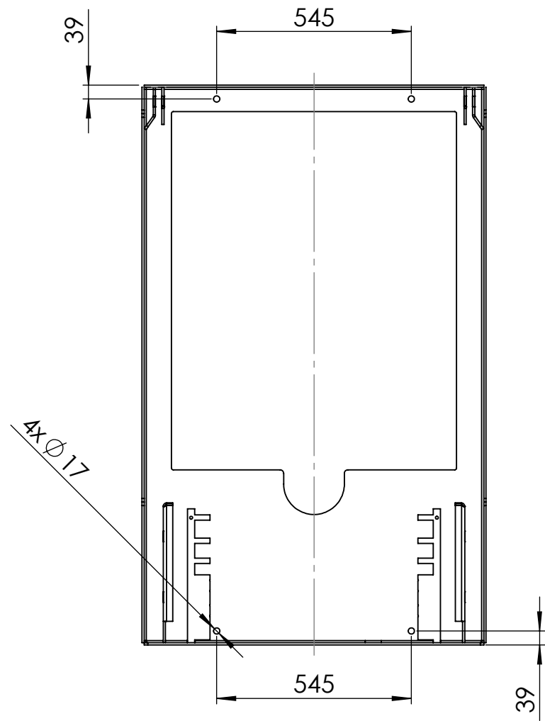
Bodenverschraubung/Bottom screwing
