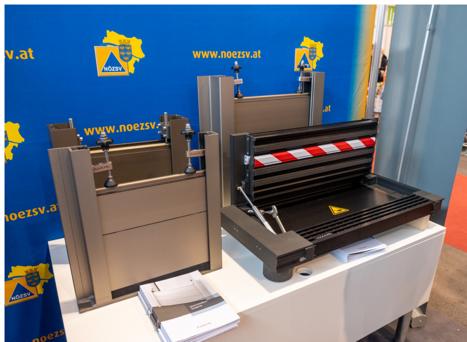
Produkte für den Hochwasserschutz der Firma Amari
