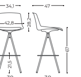
4 Metal legs stool Taburete 4 patas de metal
