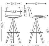
4 Wood legs stool Taburete 4 patas de madera
