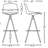
4 Metal legs stool Taburete 4 patas de metal
