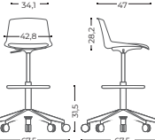
Draughtman chair Banqueta - Elevación gas
