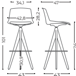
4 Wood legs stool Taburete 4 patas de madera
